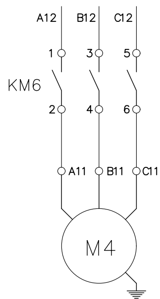
Эл. двигатель подачи
